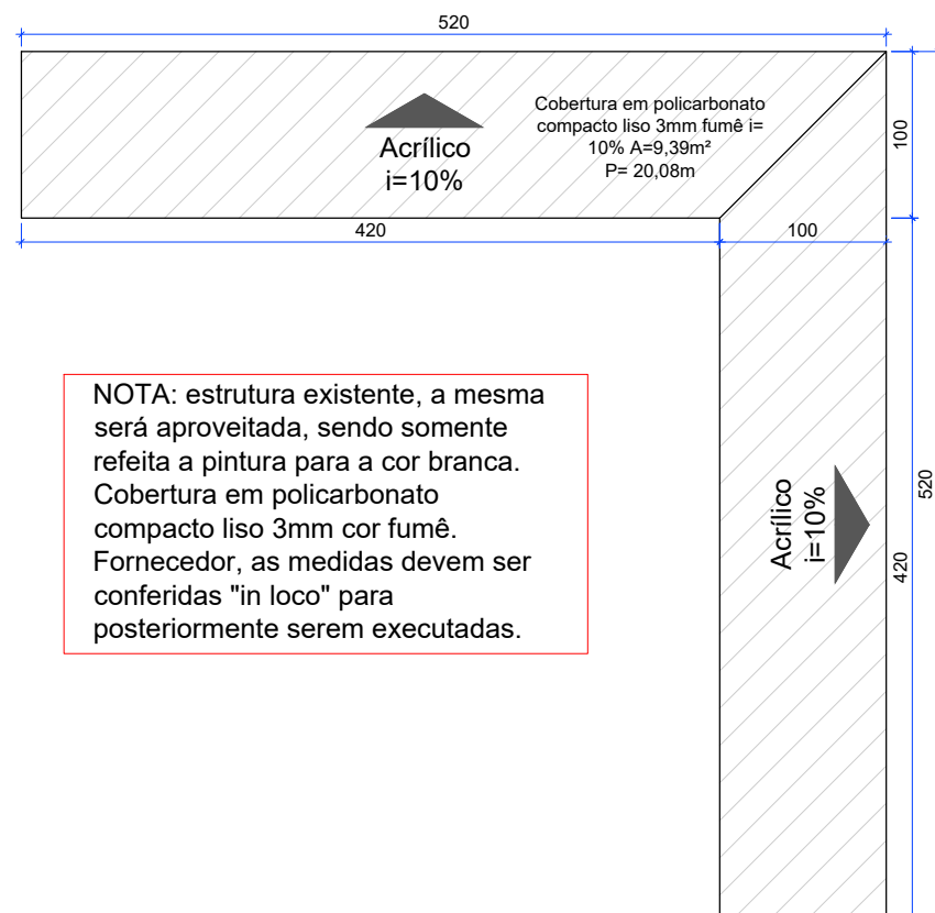
DETALHE 04- COBERTURA EXTERNA ESC.: 1:50
