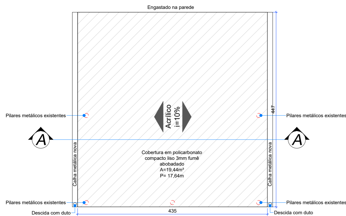
DETALHE 03- COBERTURA FRONTAL ESC.: 1:50
