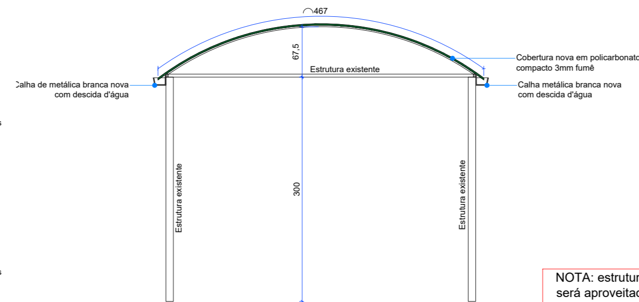
DETALHE 03- CORTE AA ESC.: 1:50
