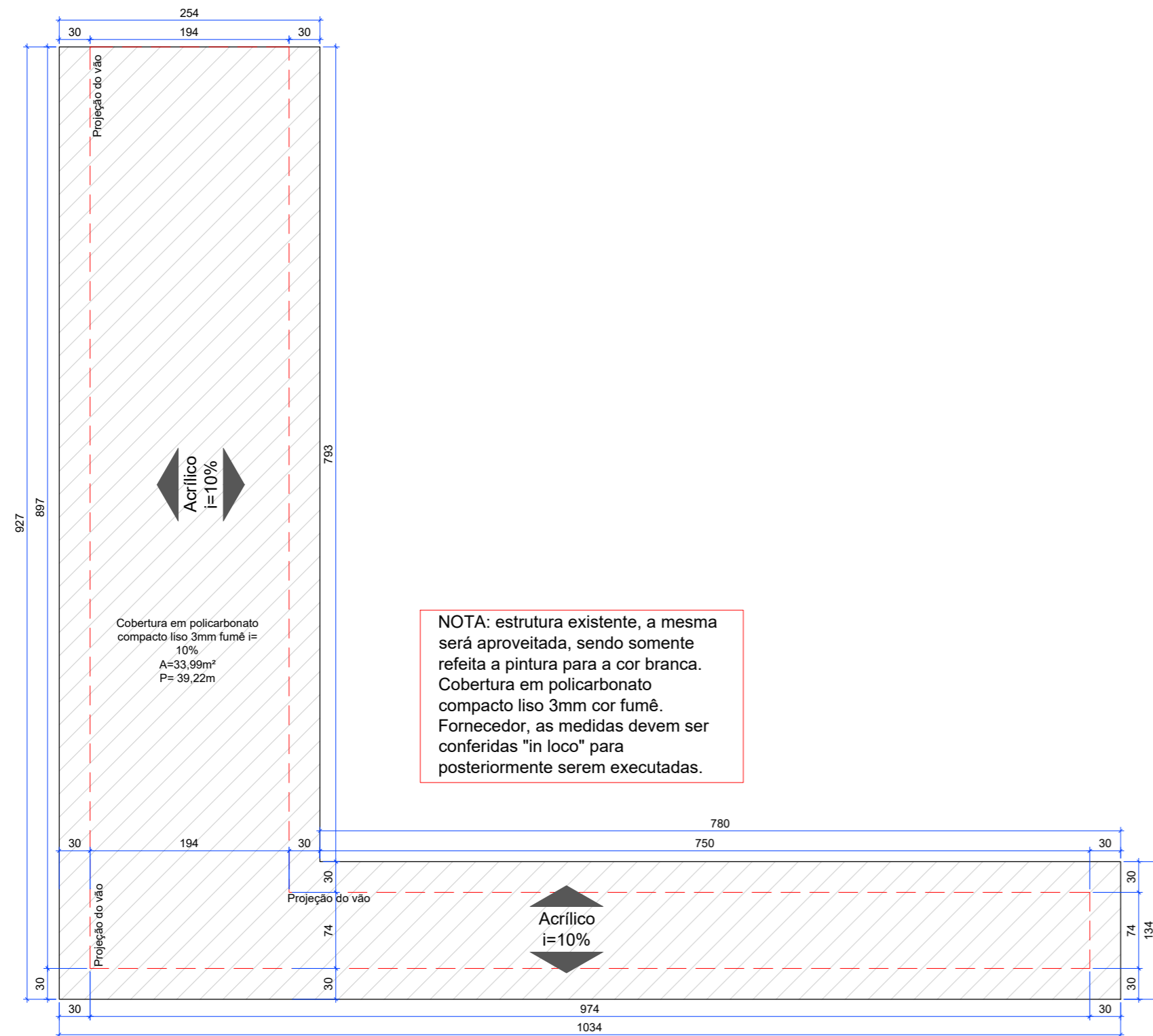
DETALHE 01- COBERTURA INTERNA ESC.: 1:50
