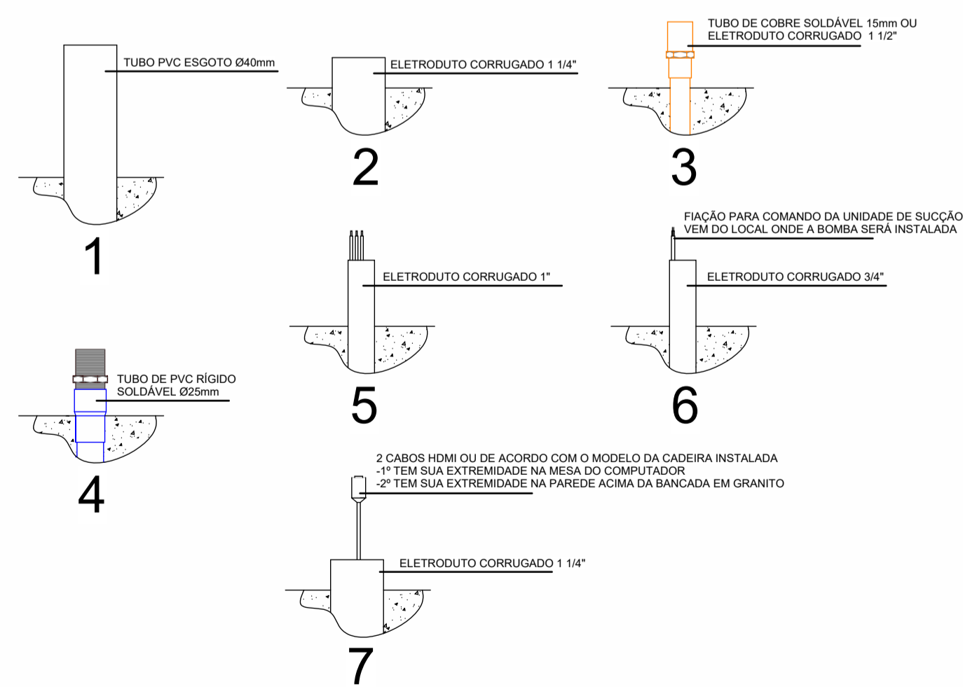
2 - DETALHE CONEXÕES CADEIRA ODONTOLÓGICA
