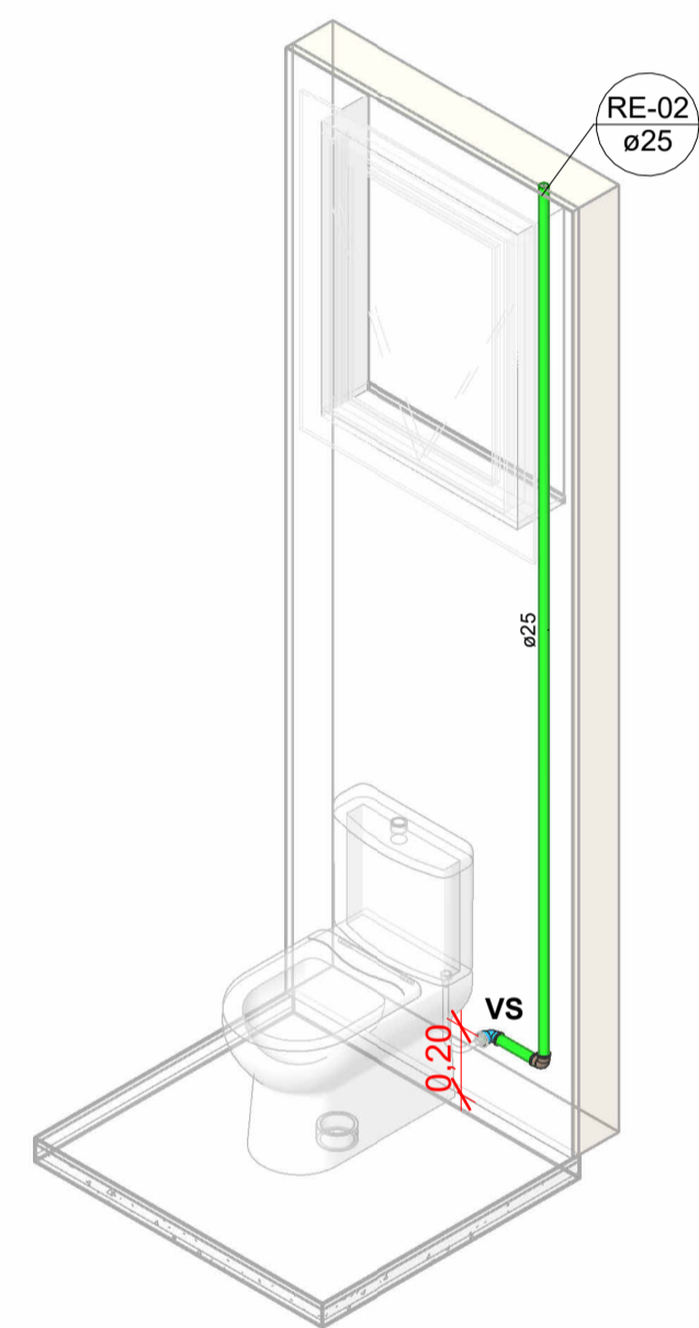
Isométricos RE-02 Escala
