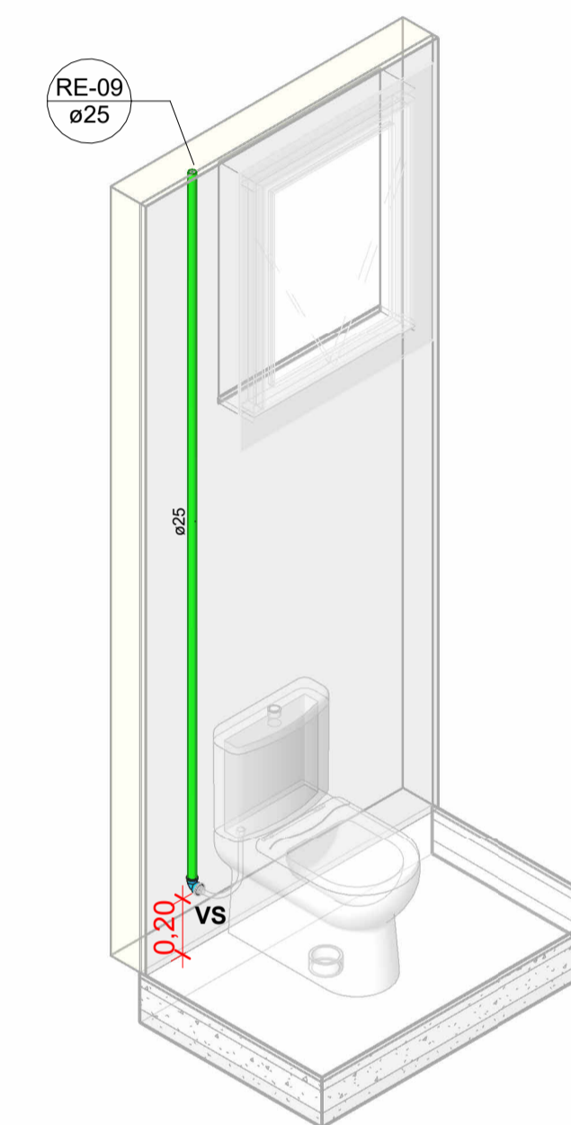
Isométricos RE-09 Escala
