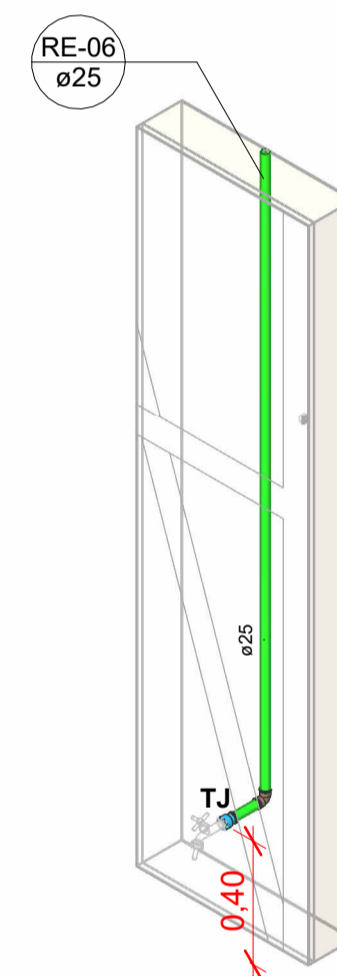
Isométricos RE-06 Escala
