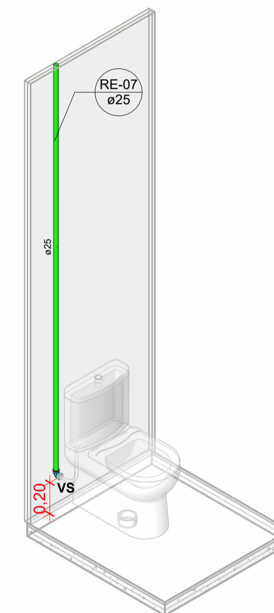
Isométricos RE-07 Escala
