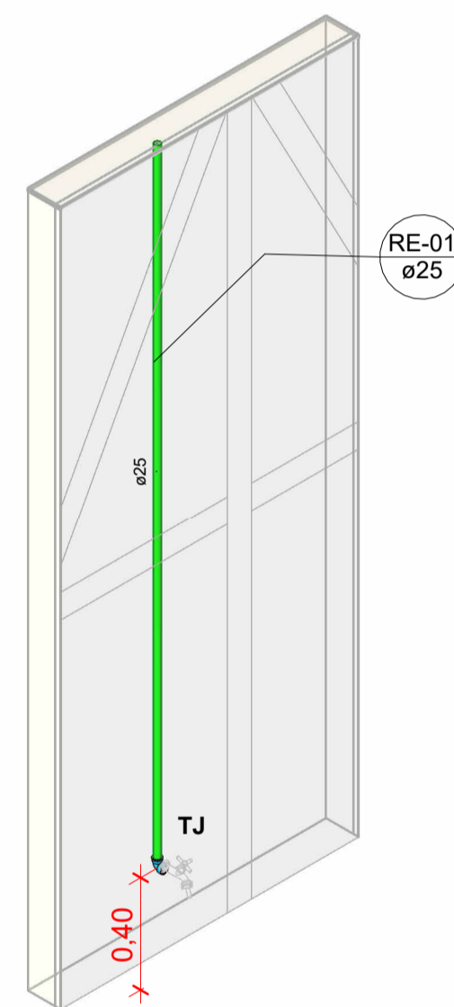
Isométricos RE-01 Escala
