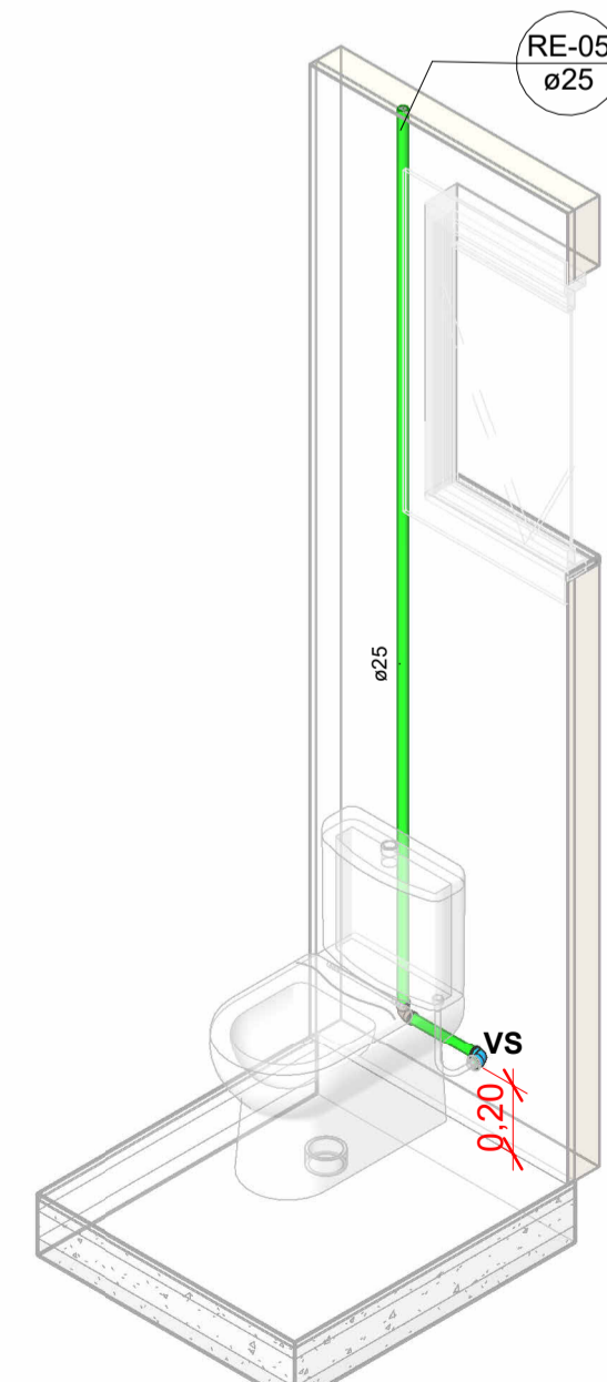
Isométricos RE-05 Escala
