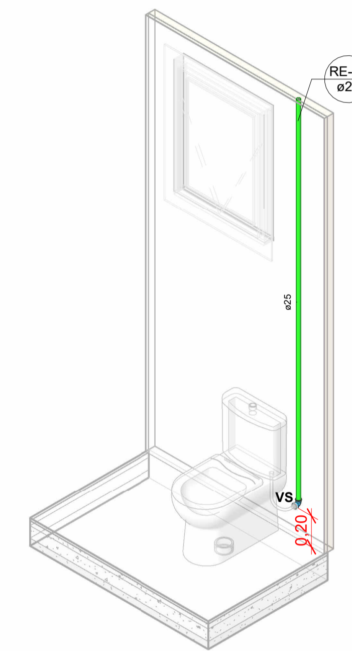
Isométricos RE-10 Escala
