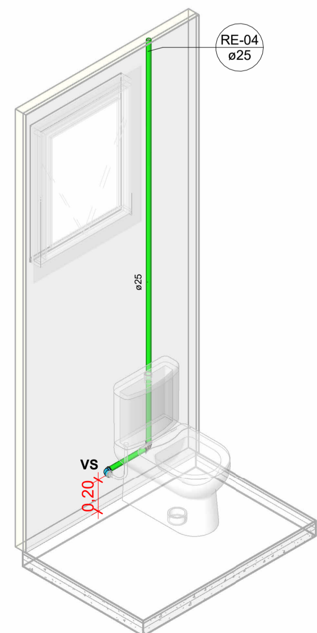
Isométricos RE-04 Escala
