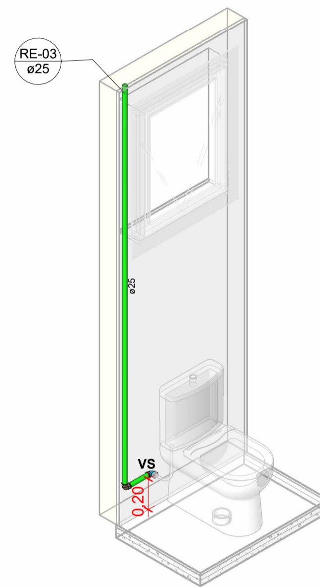
Isométricos RE-03 Escala
