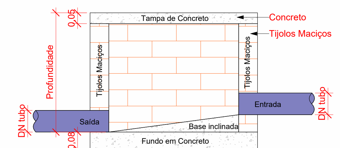
Corte lateral - Caixa de Passagem Pluvial 1 : 10 Inspeção - CP Alvenaria s/ Greiha Escala 1 : 10
