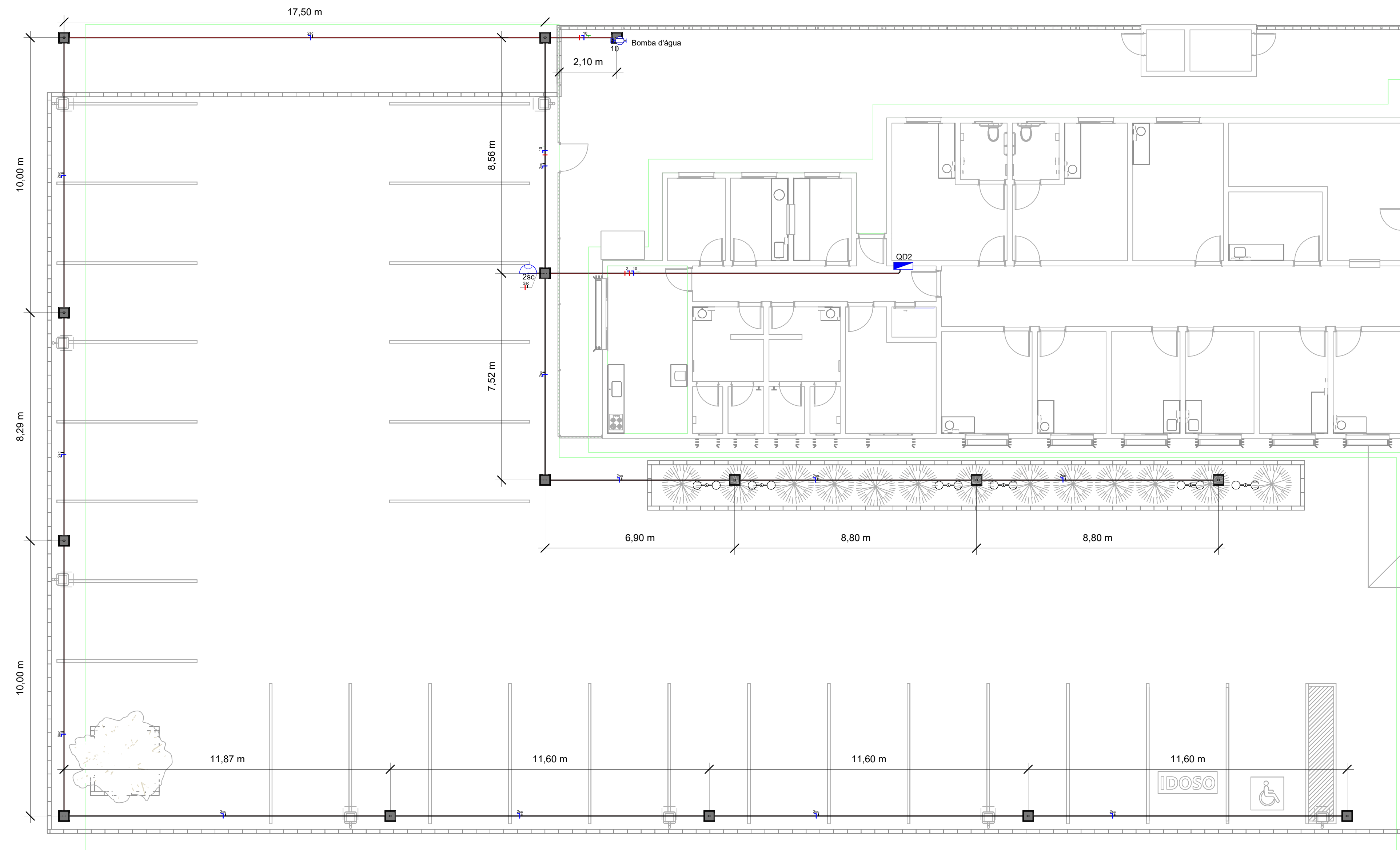
DETALHE 3 - ESTACIONAMENTO (ESCALA 1:100)
