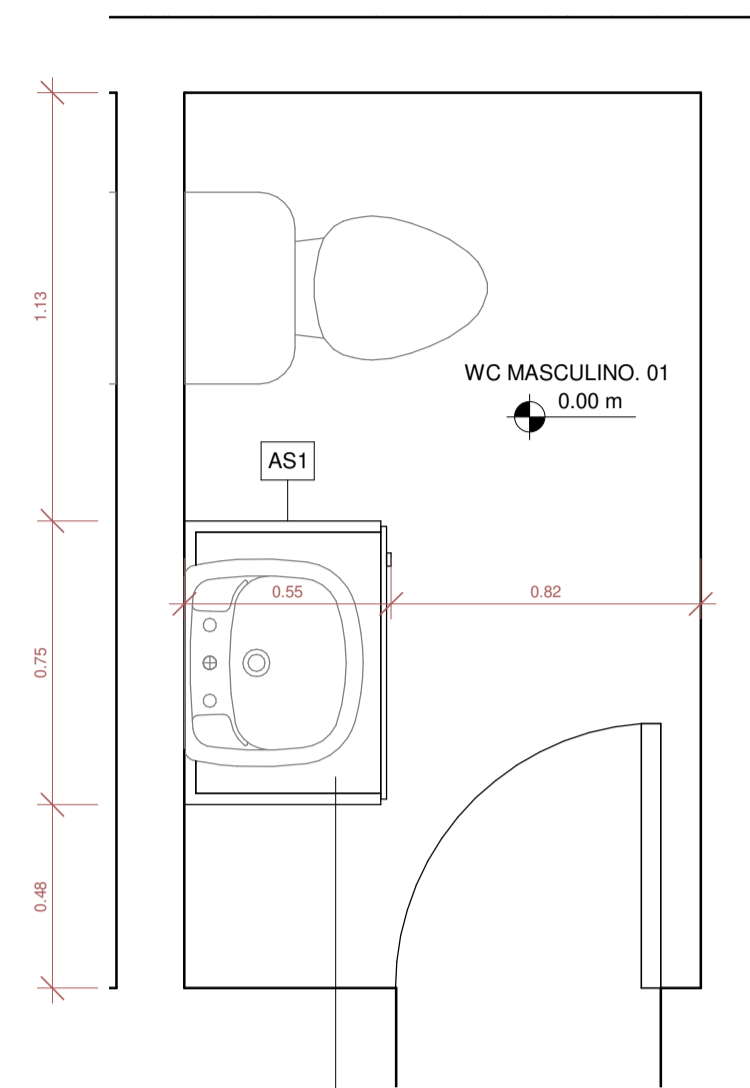
1 DET. WC MASCULINO 01 1 : 20
