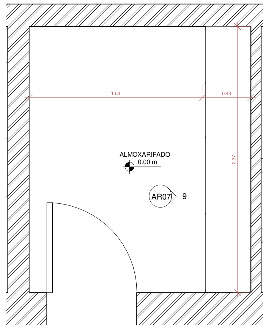
1 DET. ALMOXARIFADO 1 : 20
