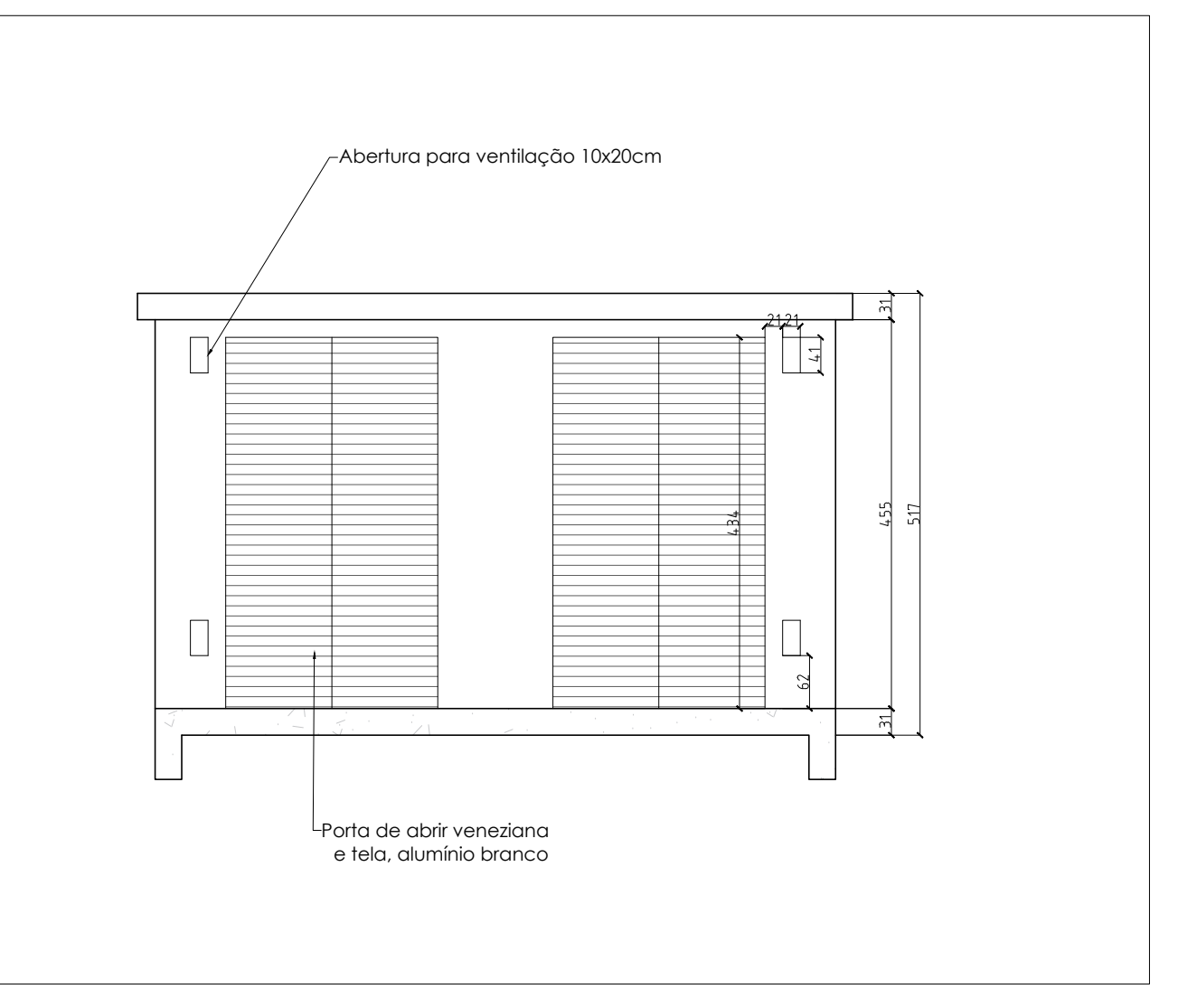
ELEVACÃO LIXEIRA
