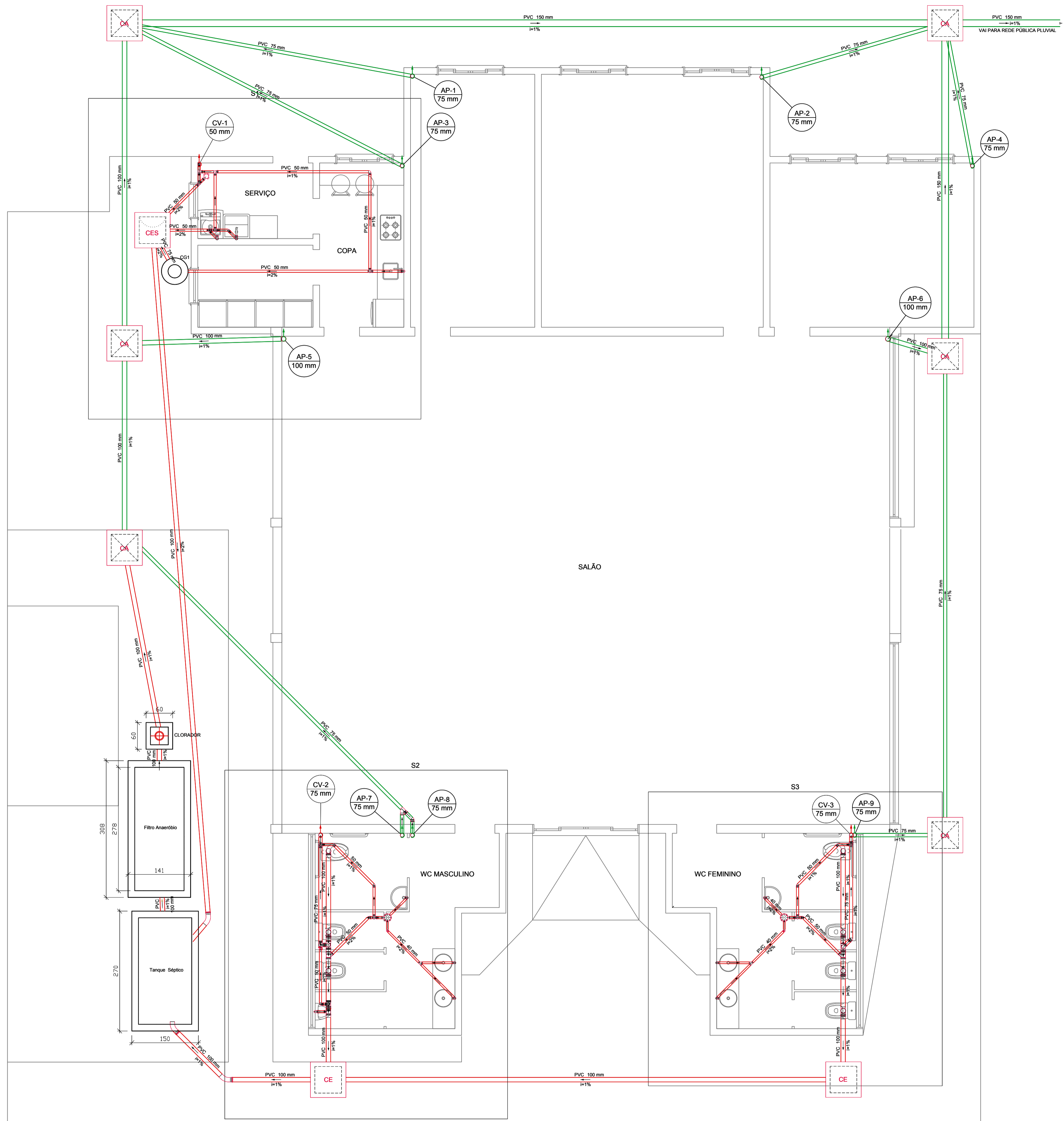
PLANTA BAIXA - PAVIMENTO TÉRREO ESCALA: 1:50
