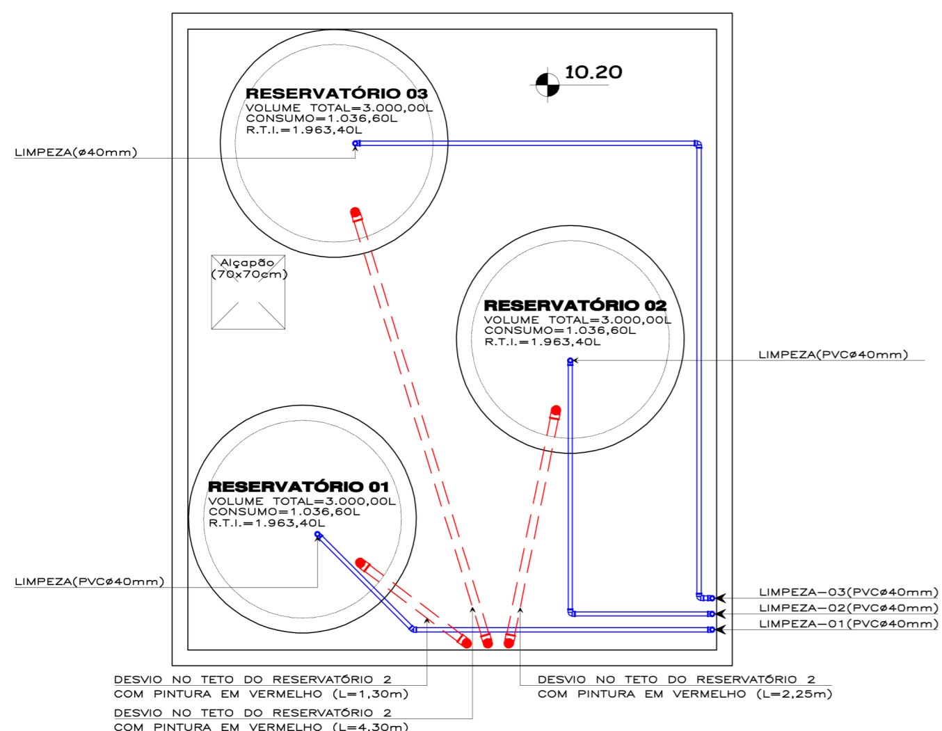
PLANTA RESERV. SUP. 1 ESCALA 1 : 50
