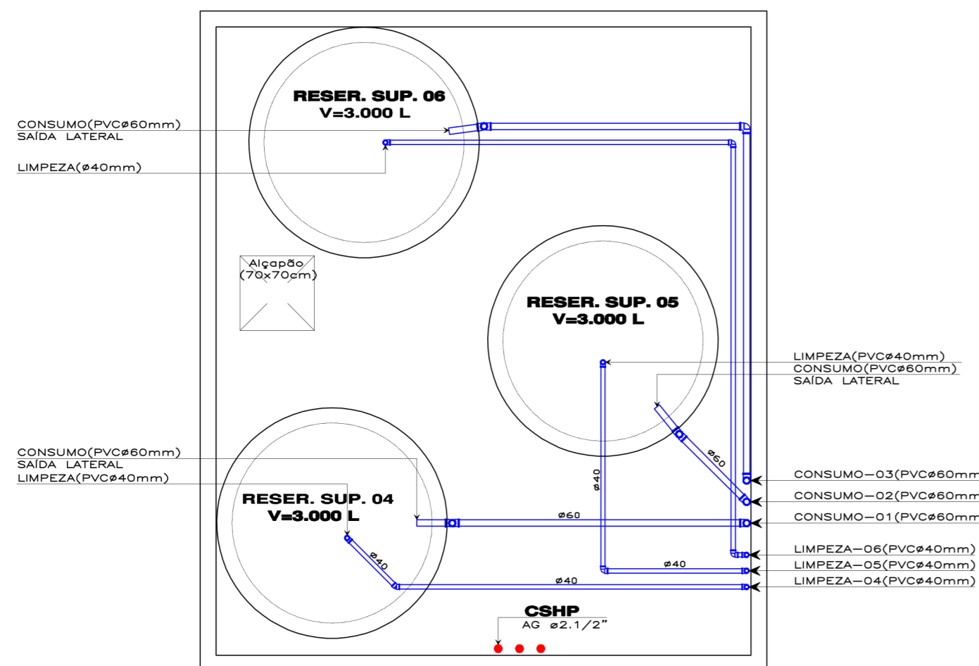
PLANTA RESERV. SUP. 2 ESCALA 1 : 50
