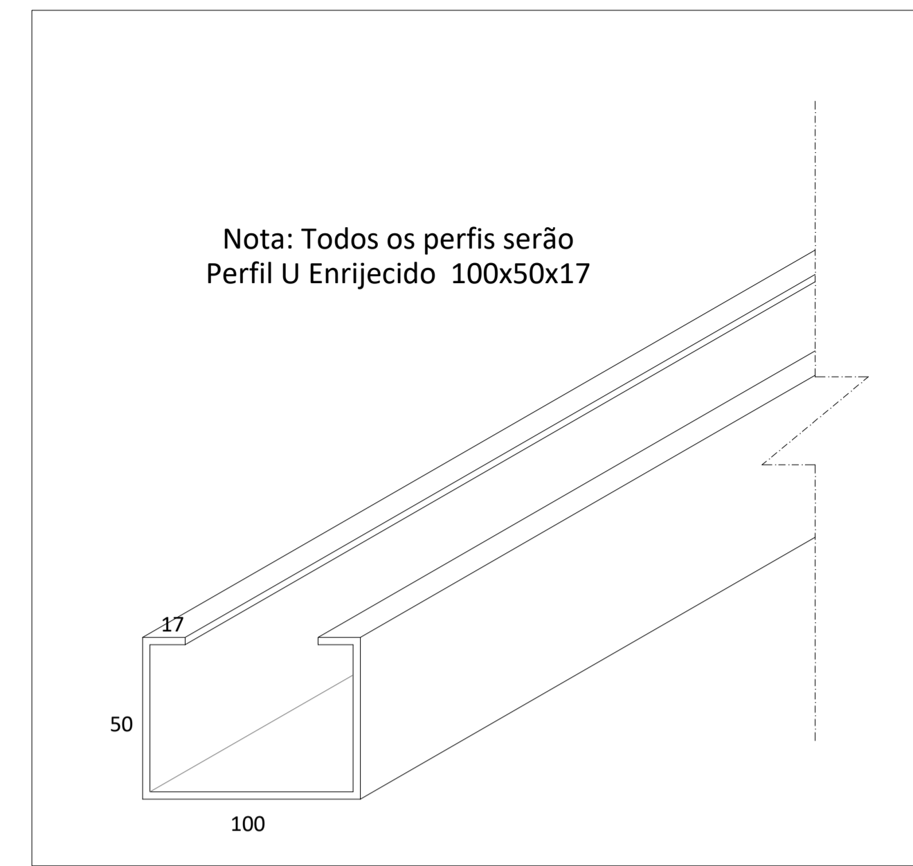
DETALHE 01 PERFIL TESOURA
