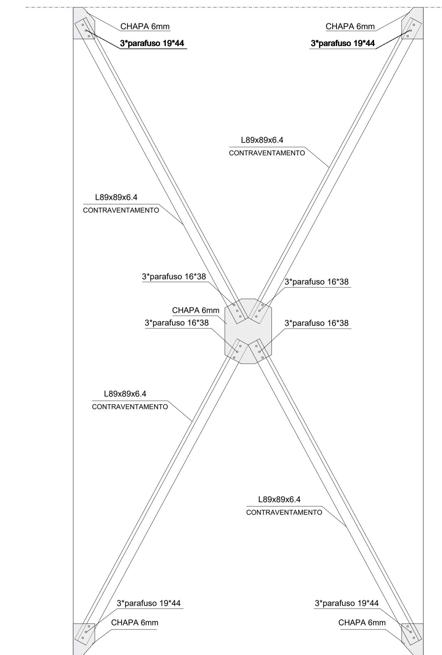
DETALHE 03 LIGAÇÕES DO CONTRAVENTAMENTO
