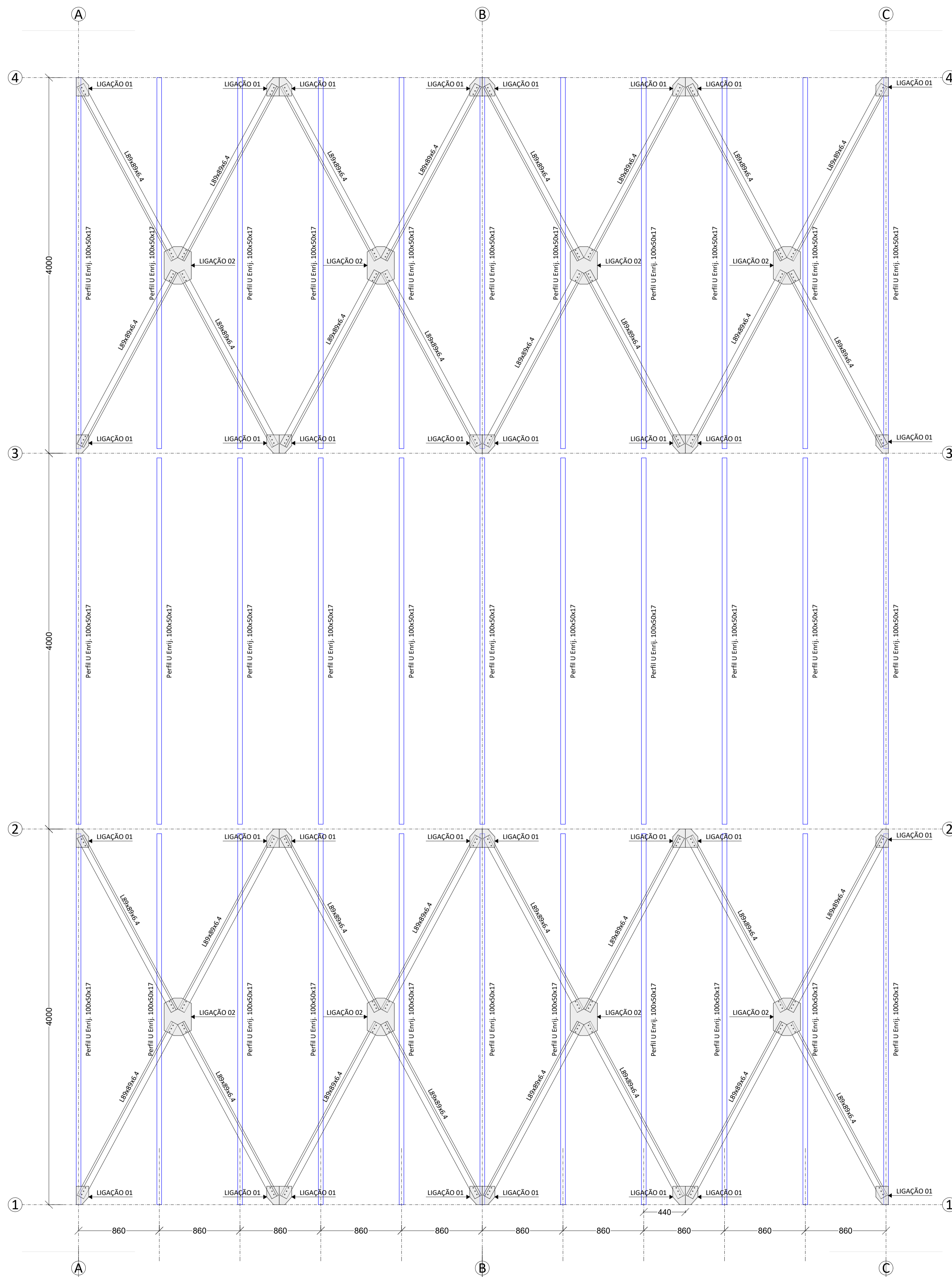
LOCAÇÃO DAS TERÇAS ESCALA: 1/25
