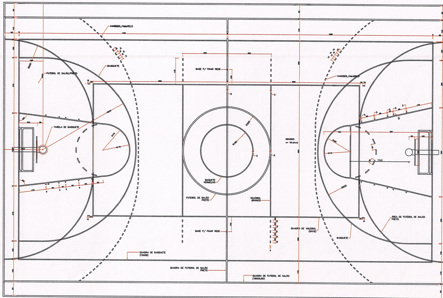
01 PLANTA - TÉCNICA
