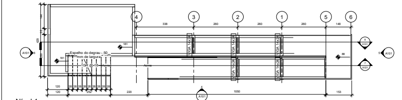
1 Nivel 1 1:50
