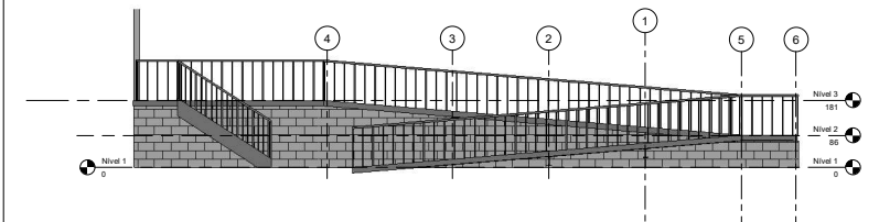
4 VISTA A 1:50
