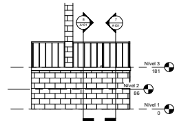
6 VISTA C 1:50
