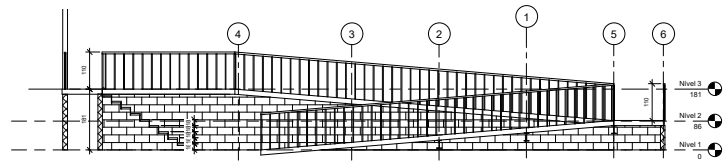
7 Corte A 1:50
