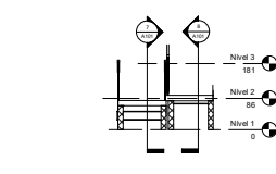
9 Corte C 1:50
