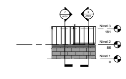
5 VISTA B 1:50
