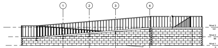
8 Corte B 1:50
