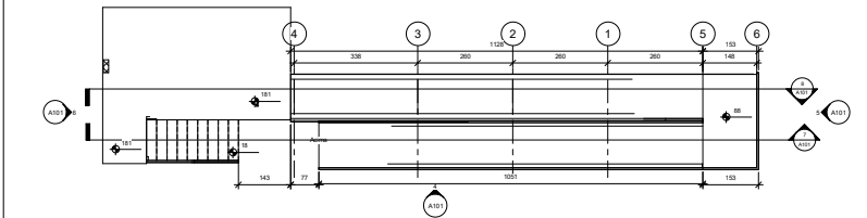
2 Nivel 2 1:50
