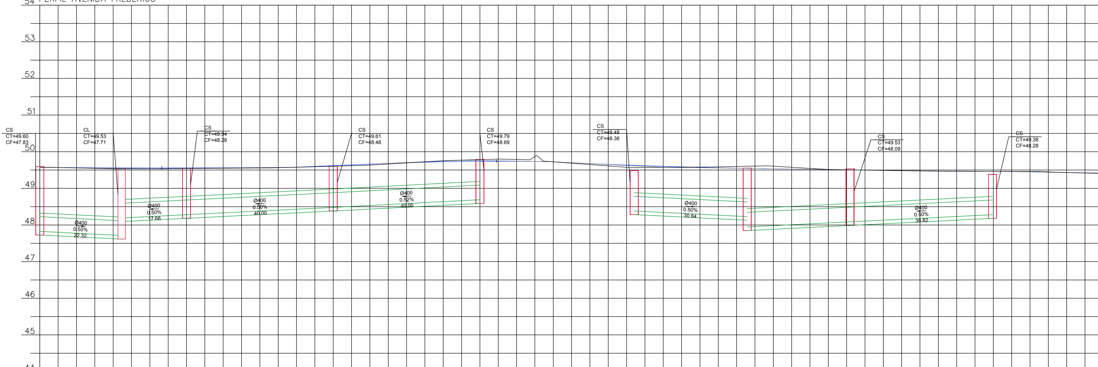
54 PERFIL AVENIDA FREDERICO
