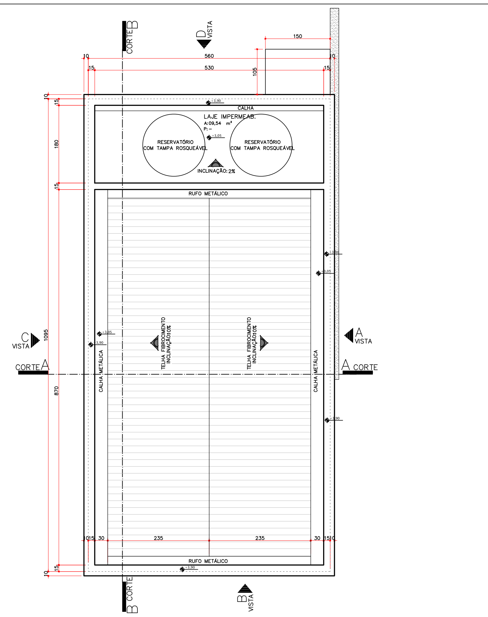
PLANTA DE COBERTURA - SANITÁRIOS E QUIOSQUE ESCALA: 1/50
